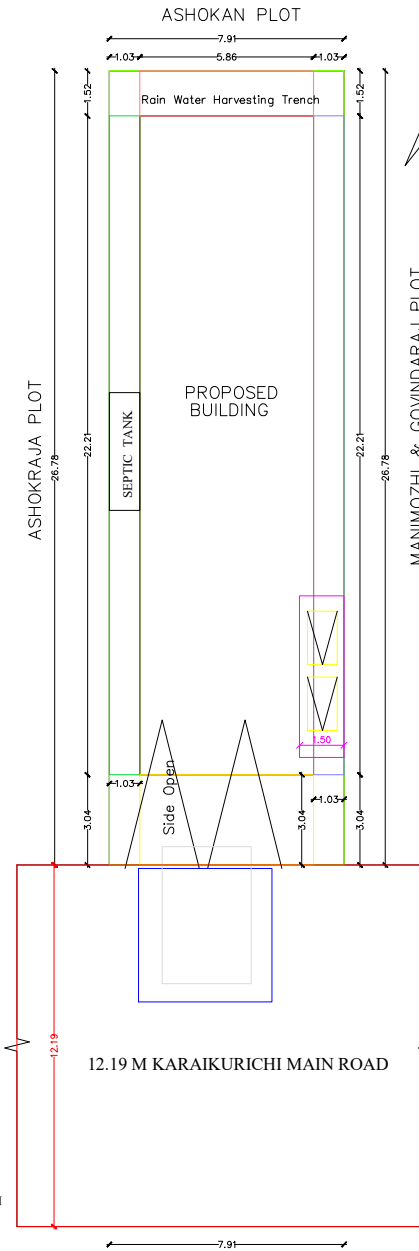
SITE PLAN SCALE : 1:100
