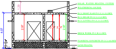
SECTION -AB
