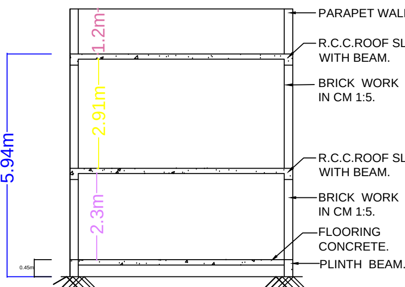
SECTION 'A'
