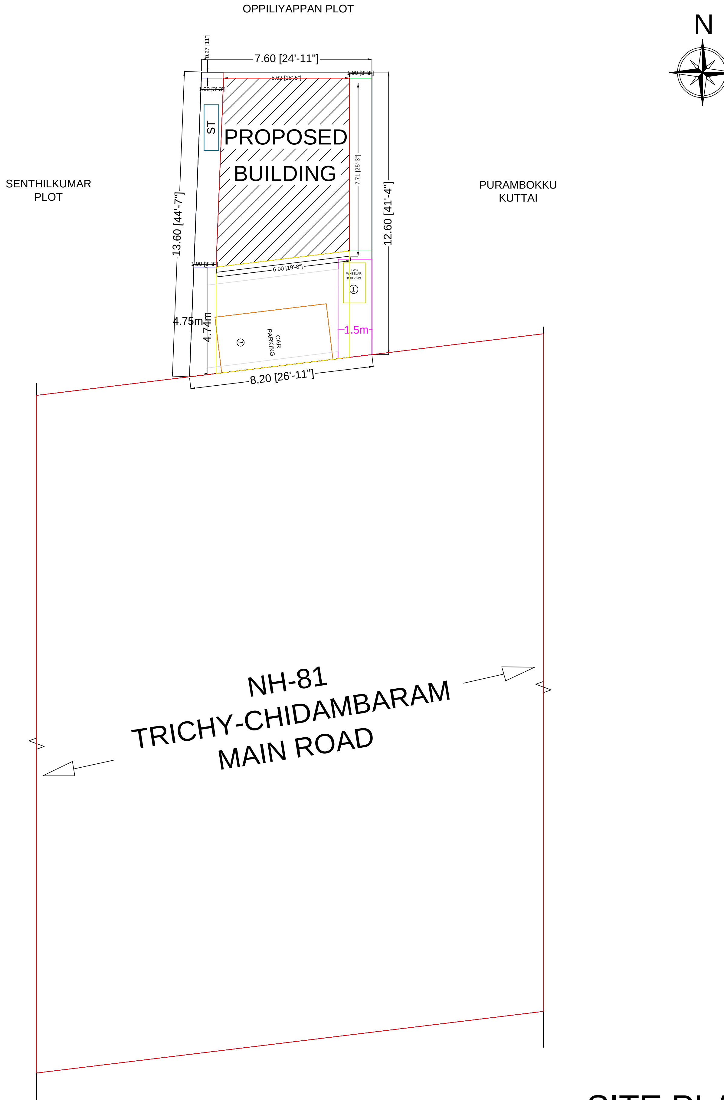
SITE PLAN (Scale 1:400)
