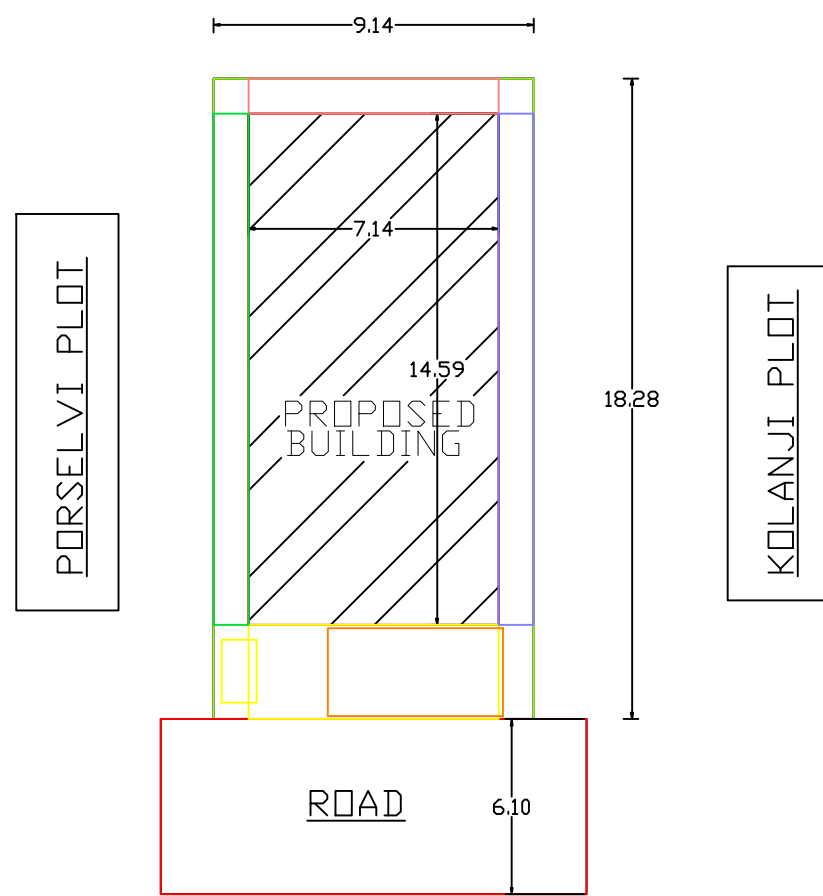
SITE PLAN 1:100 SCALE
