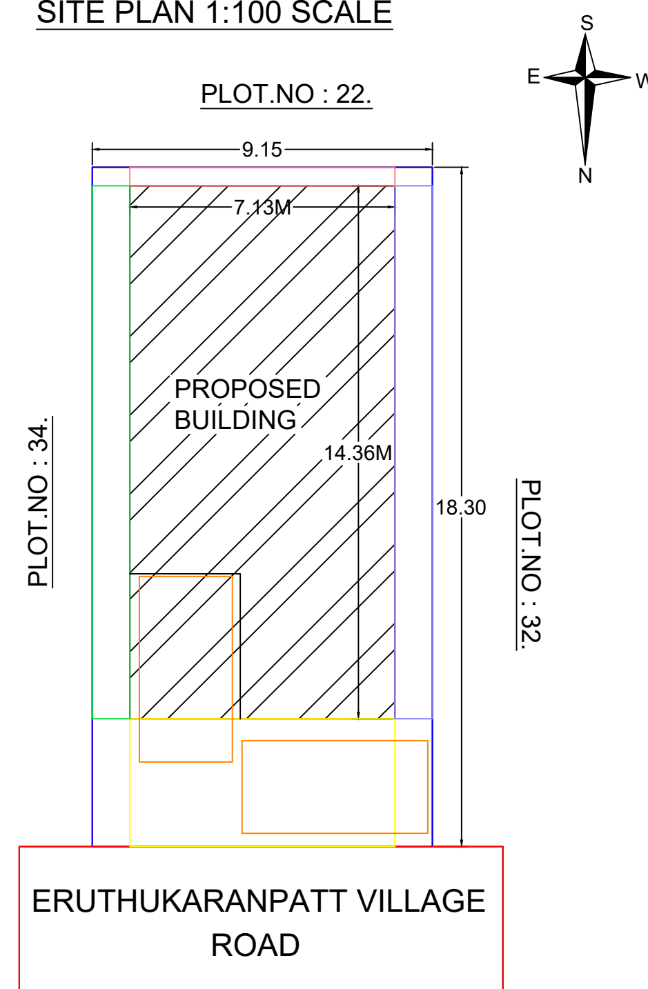
SITE PLAN 1:100 SCALE
