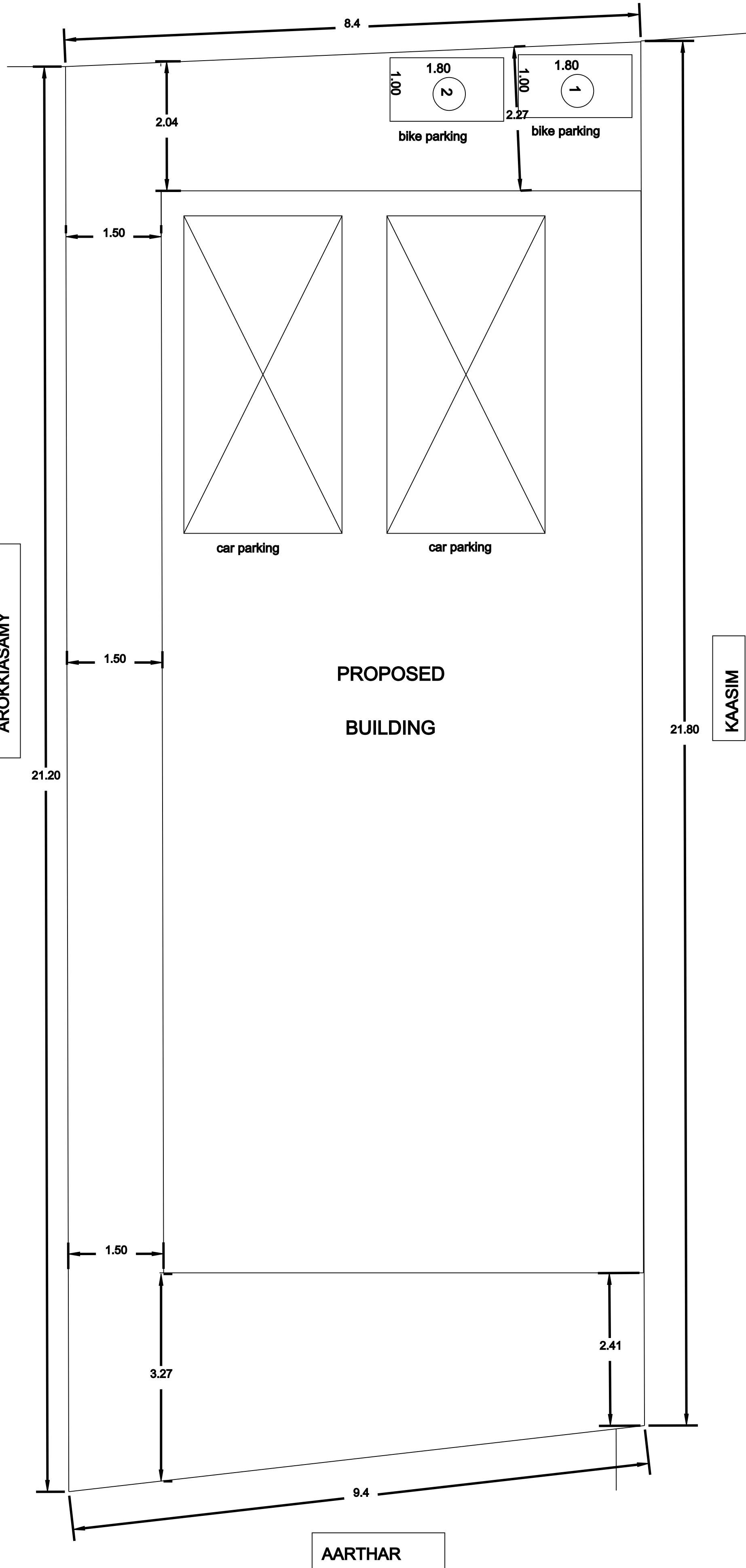
SITE PLAN1:100
