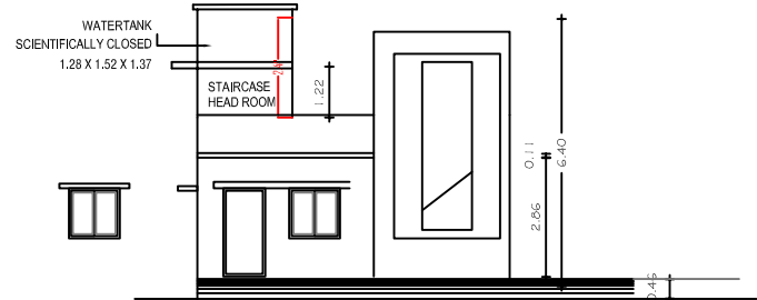
ELEVATION
