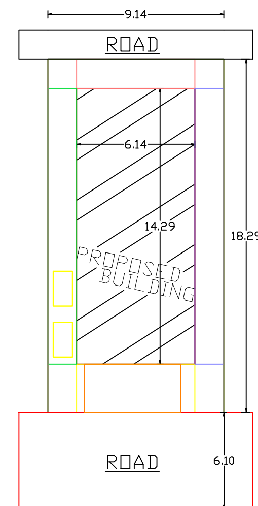
SITE PLAN 1:100 SCALE
