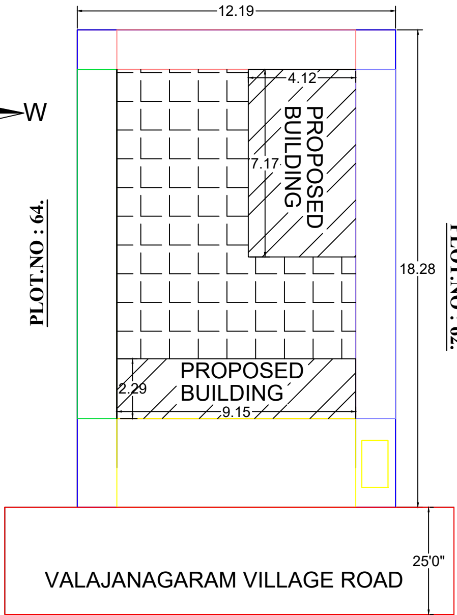
SITE PLAN 1:100 SCALE PLOT.NO : 66.
