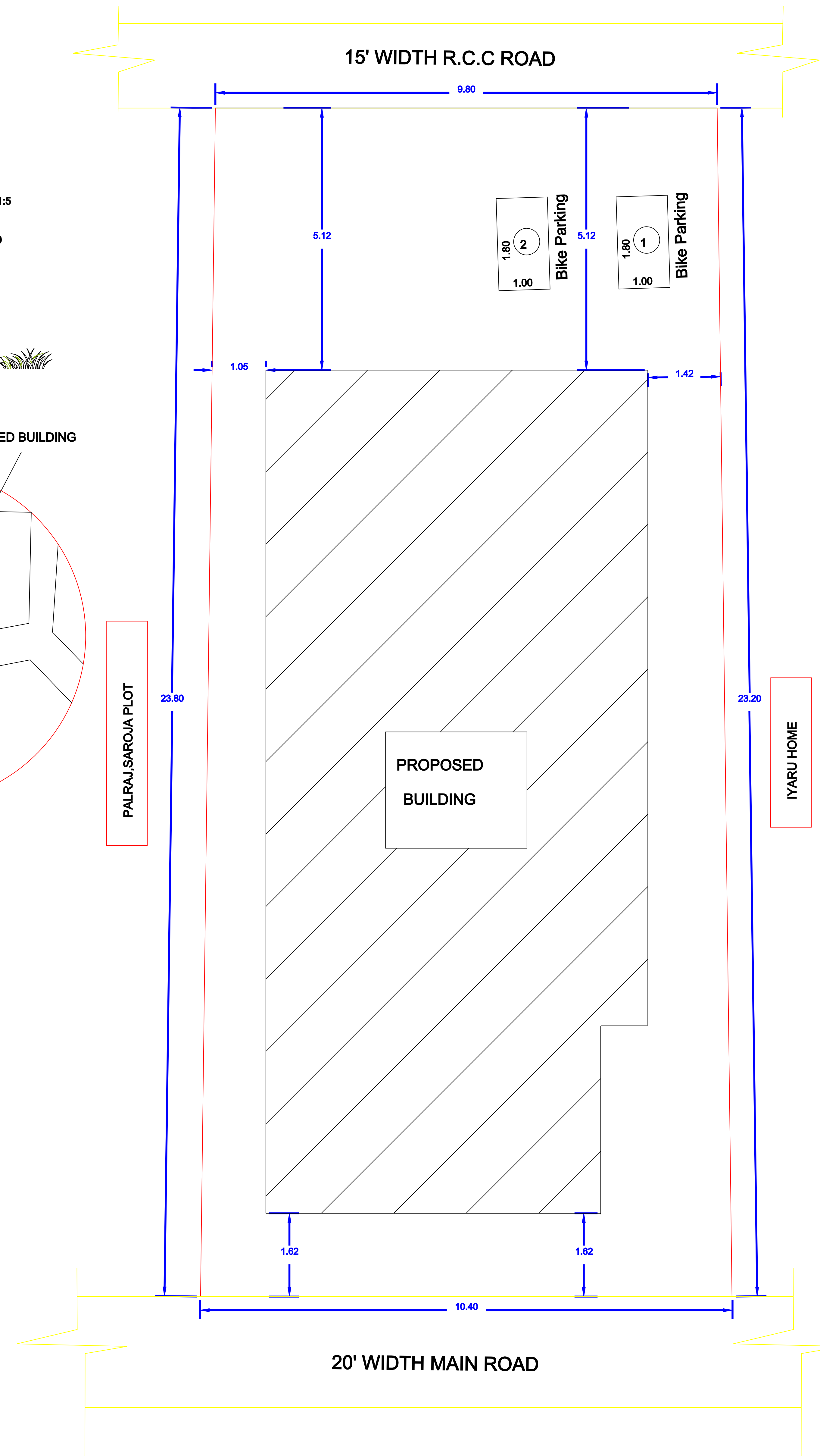
SITE PLAN1:100
