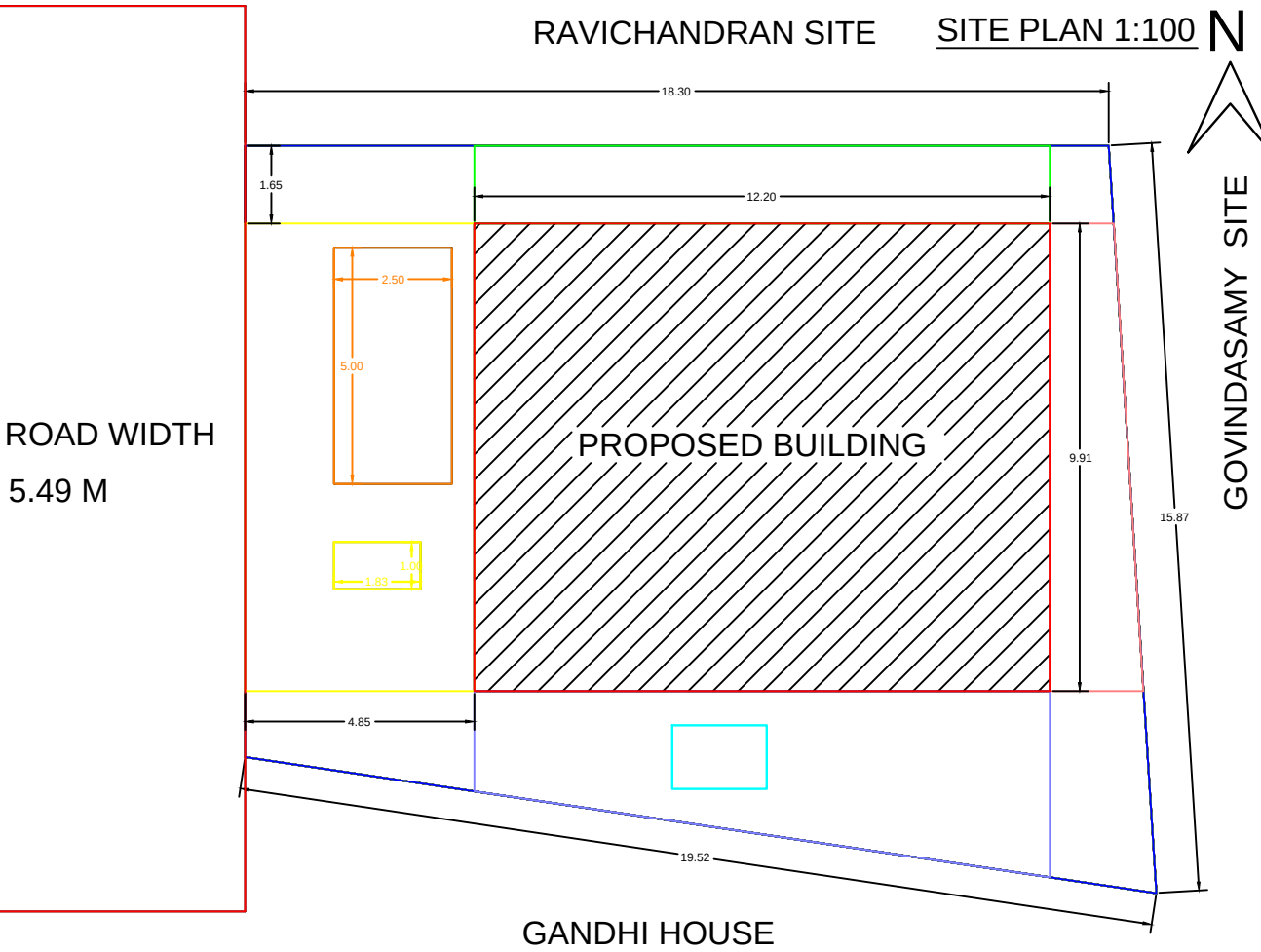
SITE PLAN 1:100
