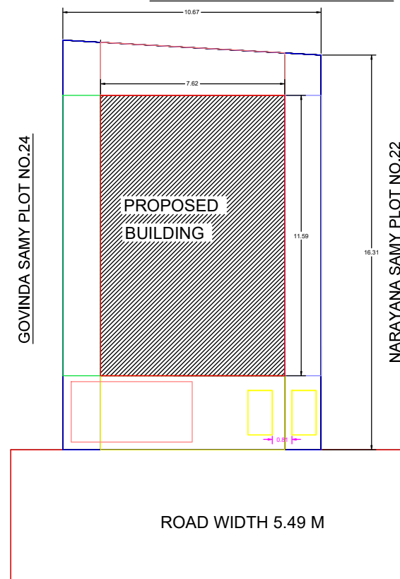
SITE PLAN 1:100 PALAMALAI CHINNA AMMAL SITE
