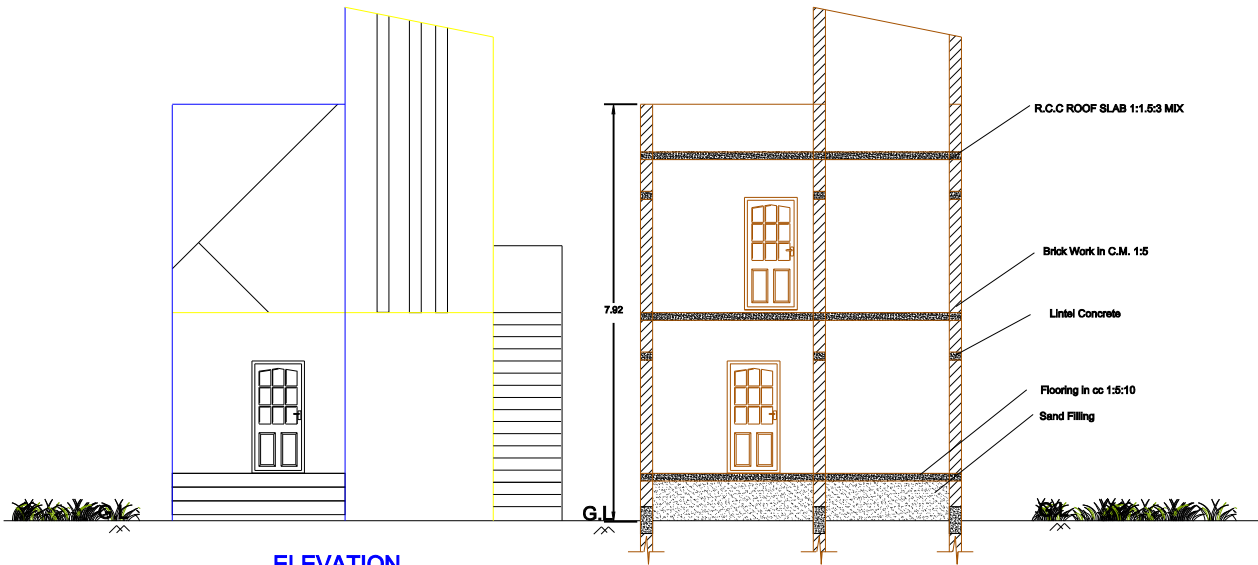
ELEVATION
