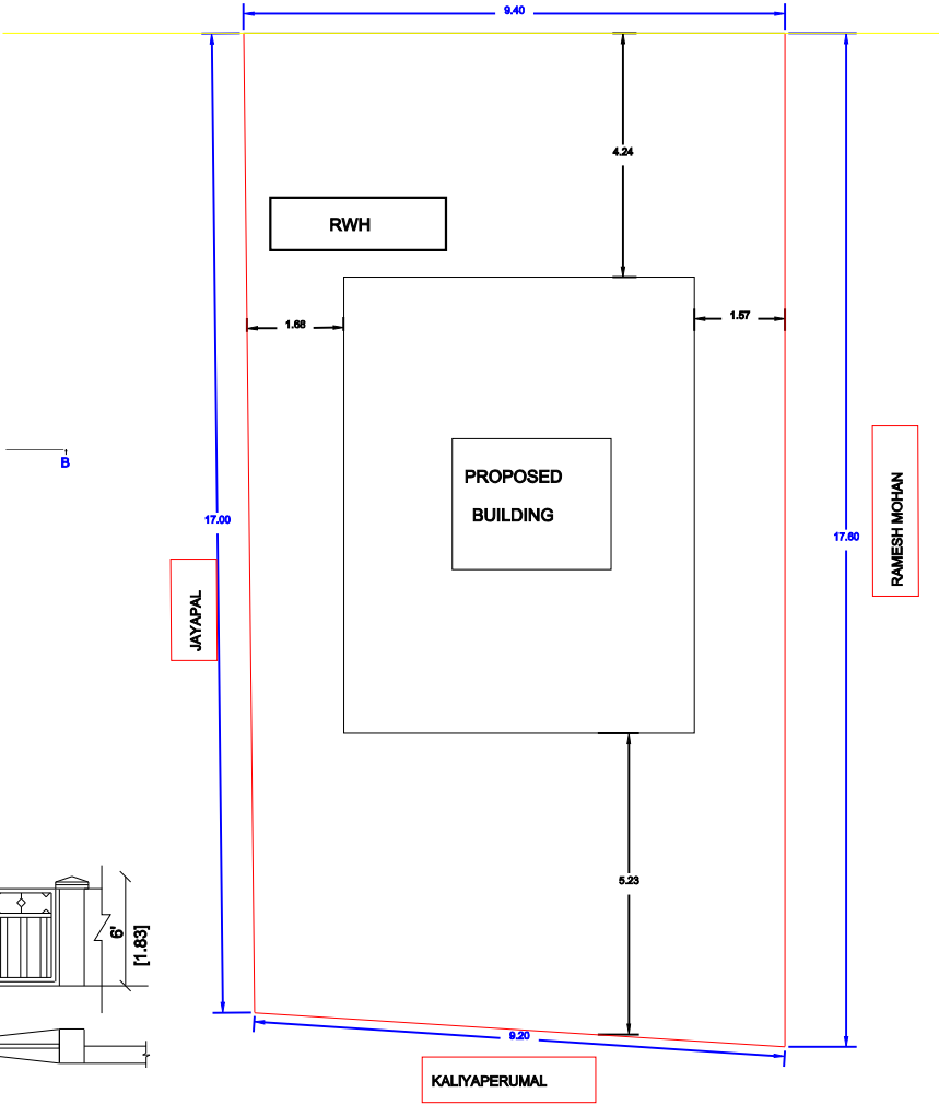
SITE PLAN 1:100
