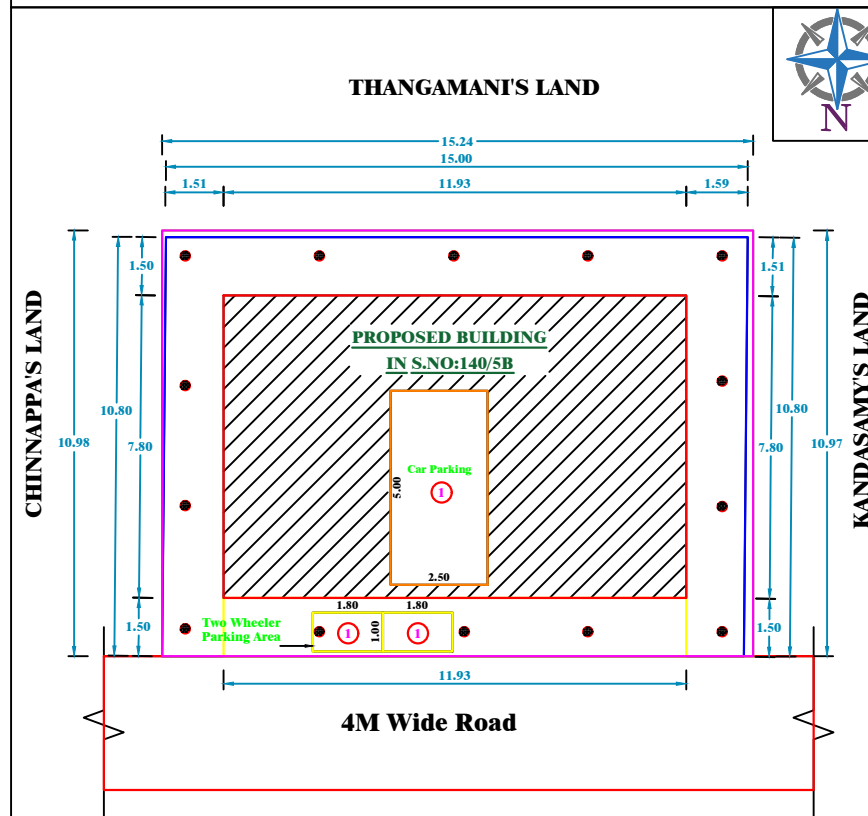
SITE PLAN-SCALE(1:100)
