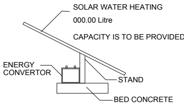
LONGITUDINAL SECTION
