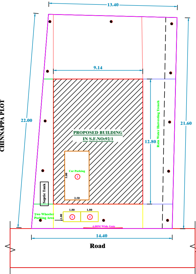
SITE PLAN-SCALE(1:100)
