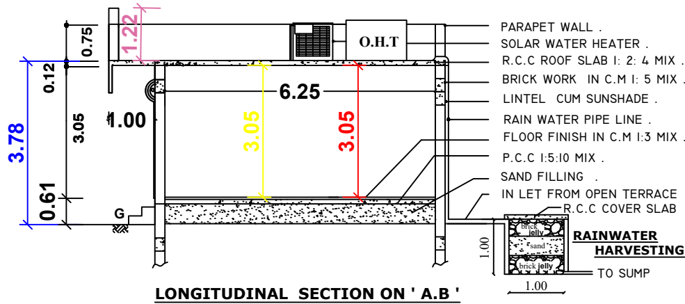
LONGITUDINAL SECTION ON 'A.B'
