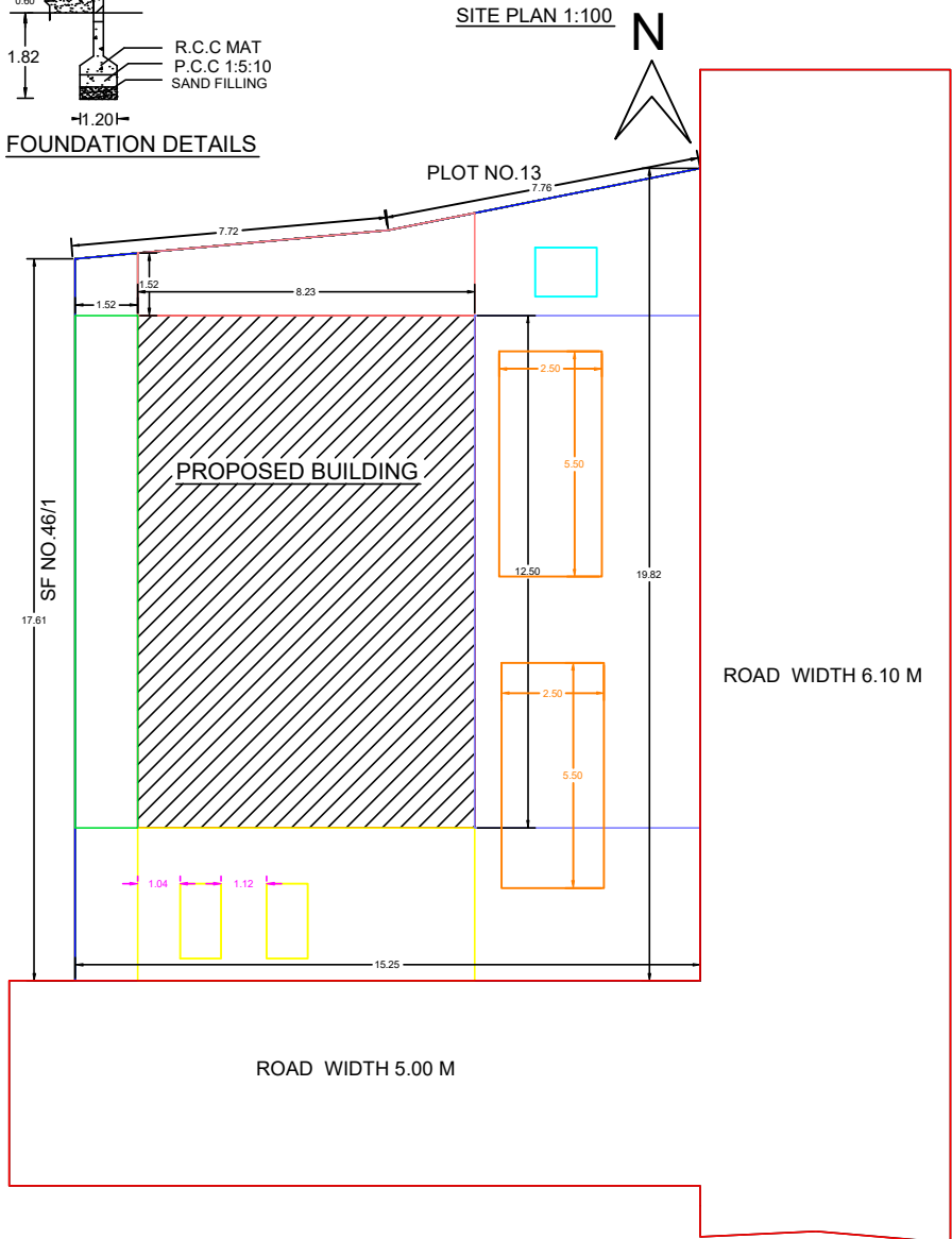
SITE PLAN 1:100
