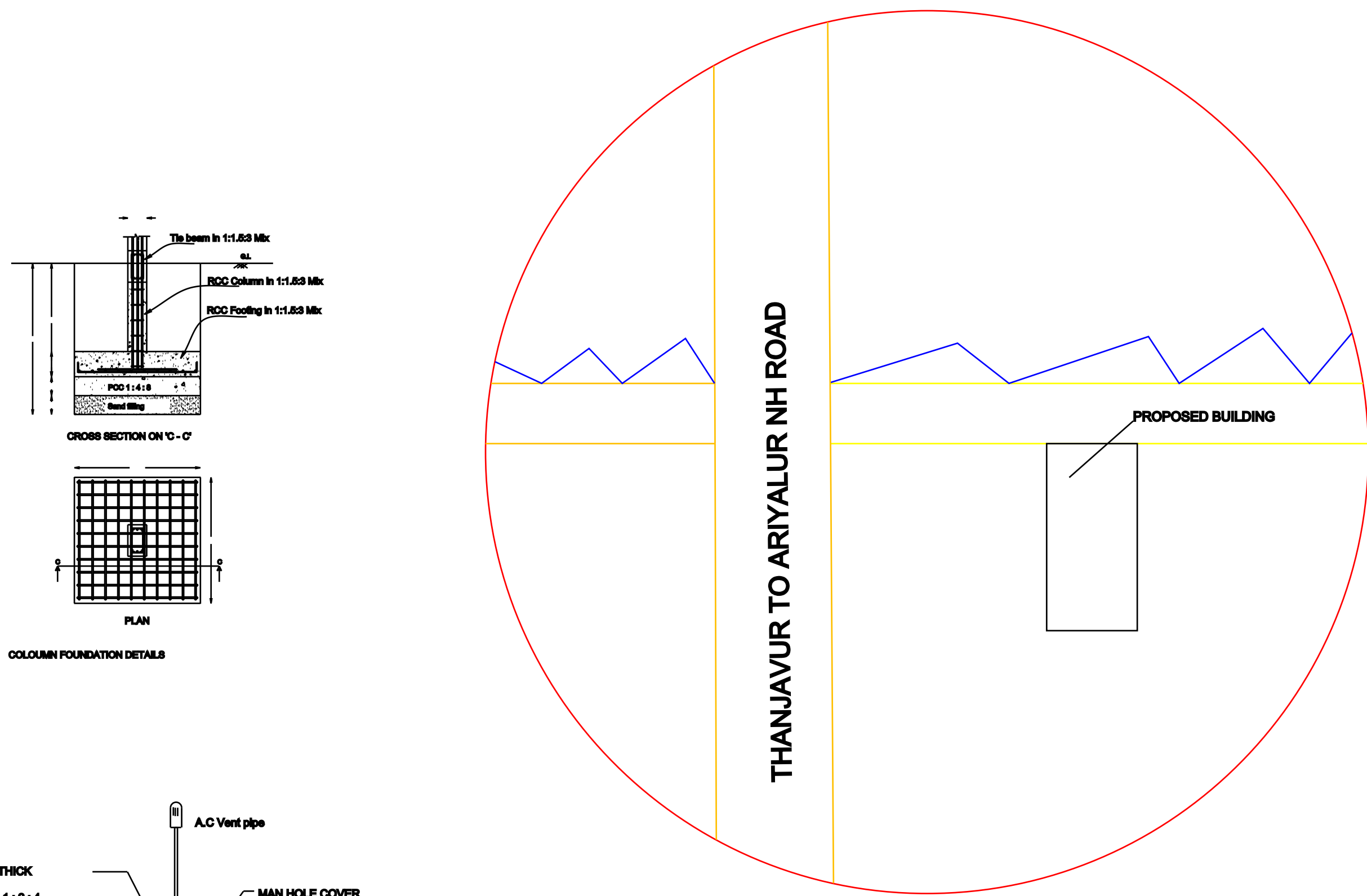
KEY PLAN (NON SCALE)
