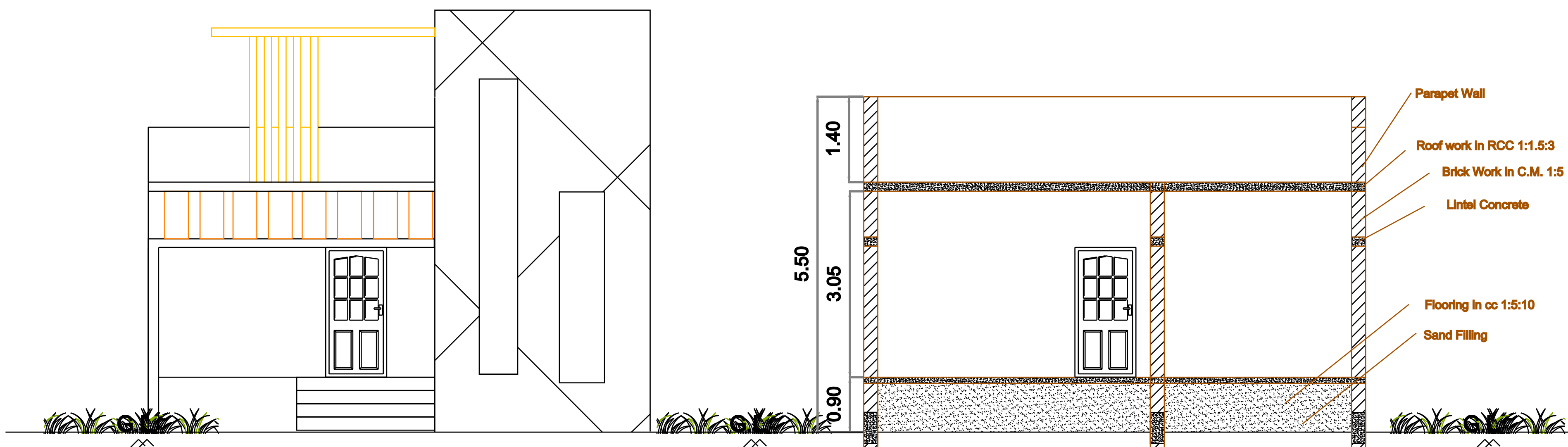
ELEVATION
