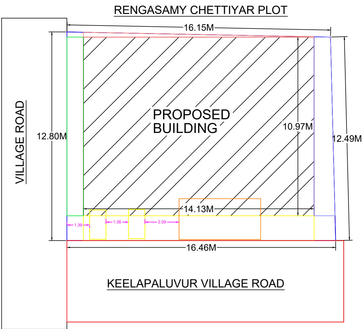
SITE PLAN 1:100 SCALE
