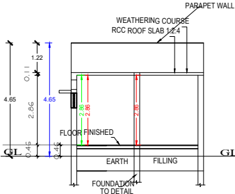
SECTION A.B
