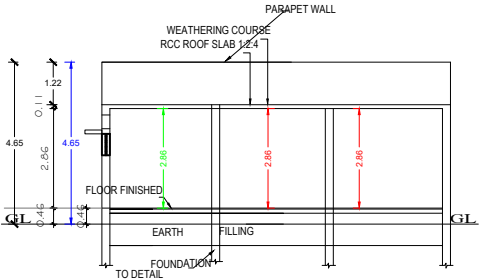
SECTION A.B
