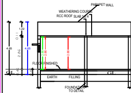
SECTION A.B
