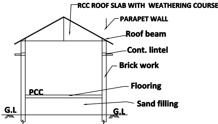
SECTION -AB
