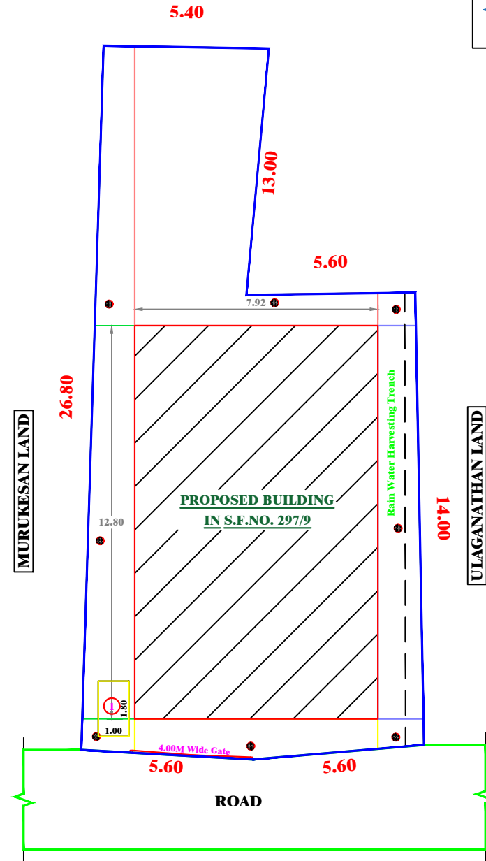
SITE PLAN-(SCALE1:500)
