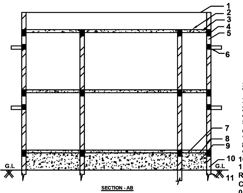
SECTION - AB
