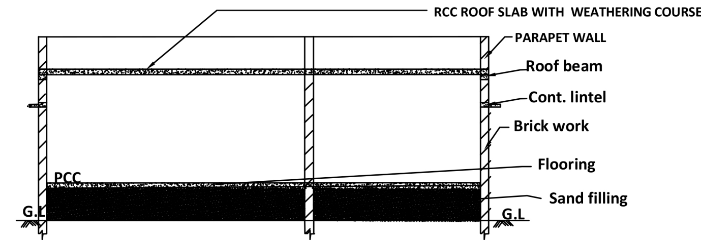
SECTION -AB
