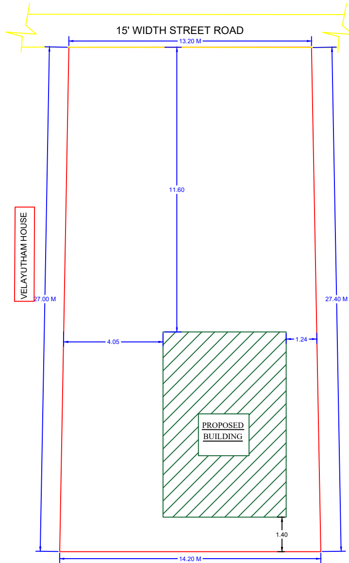
SITE PLAN 1:100
