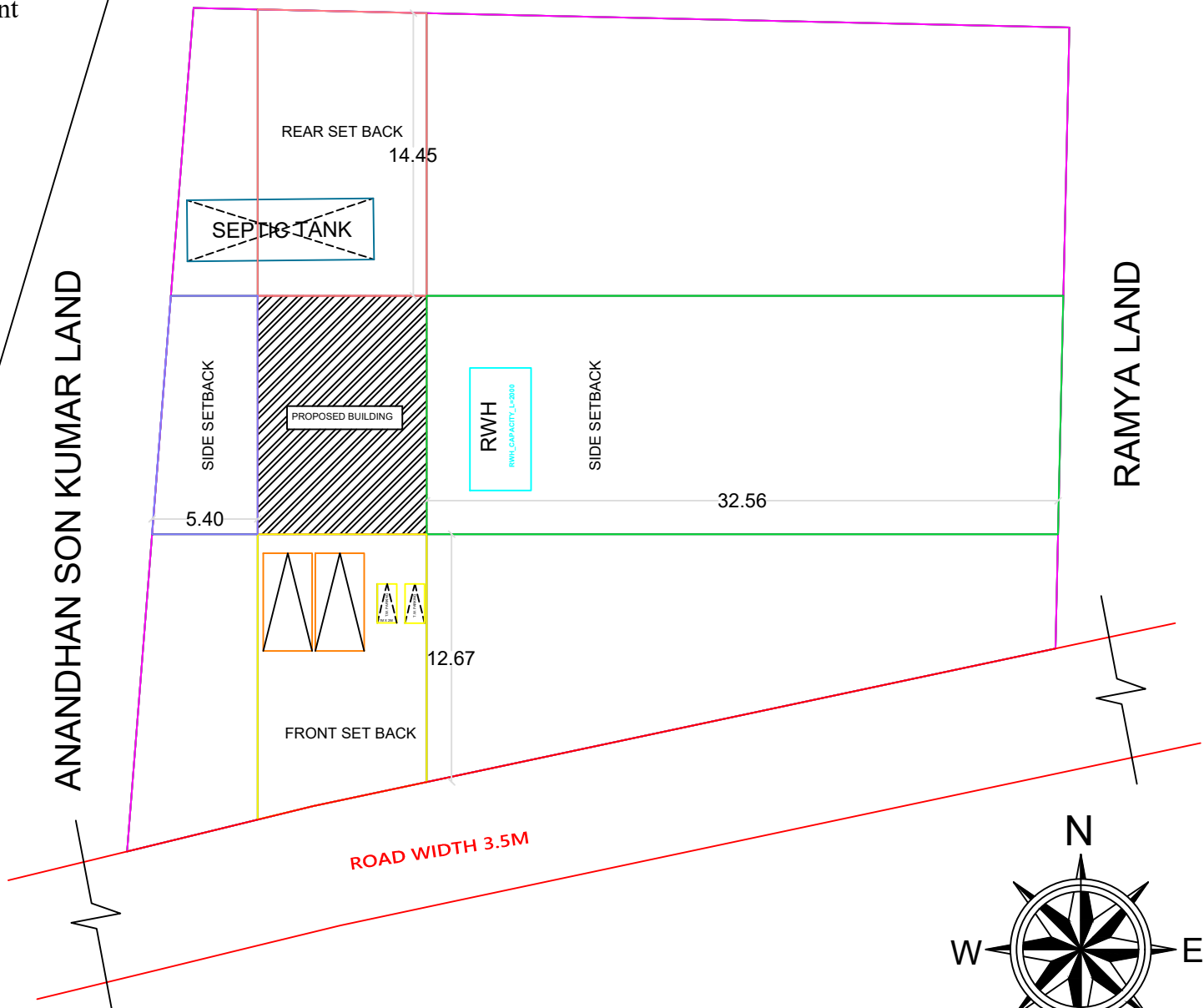
SITE PLAN 1:100
