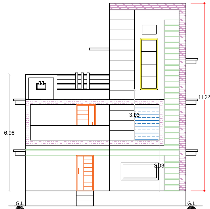
ELEVATION
