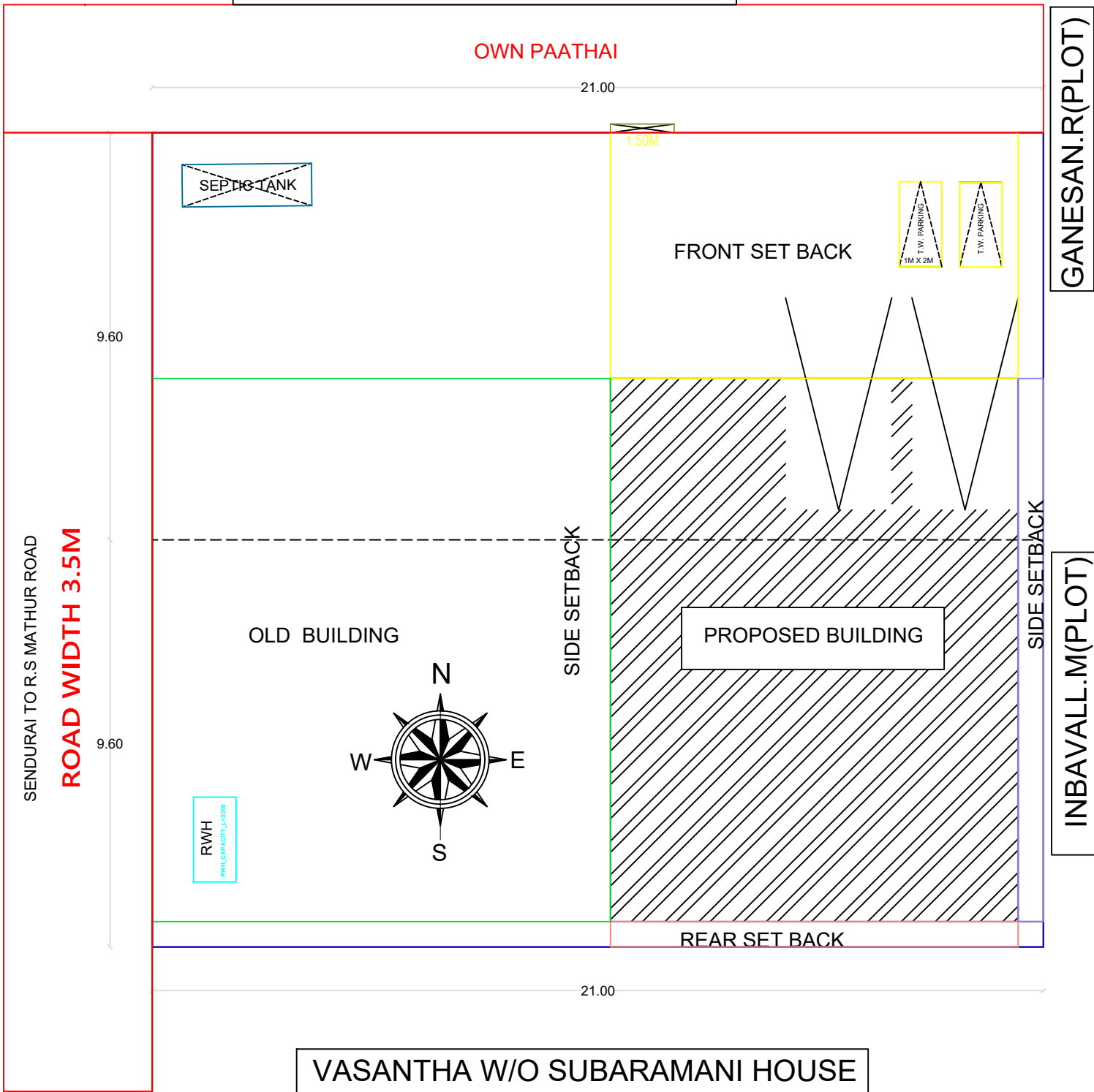
SITE PLAN 1:100 SCALE
