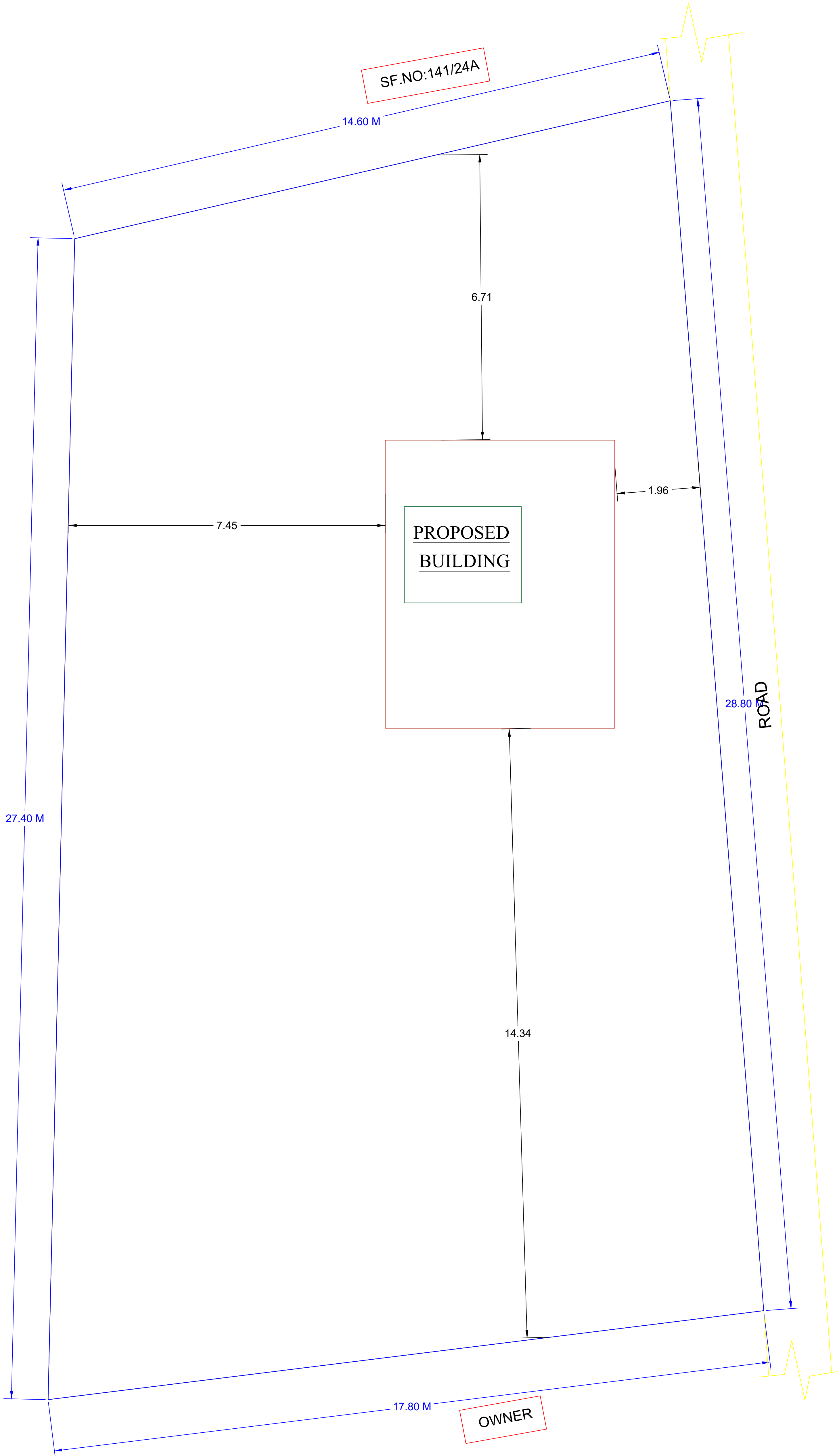
SITE PLAN 1:100
