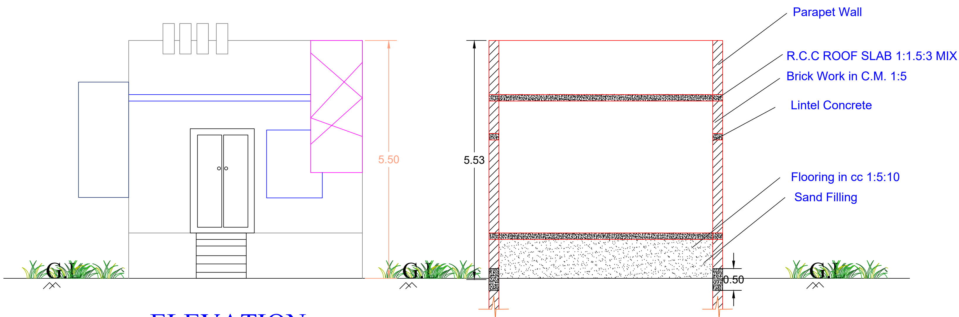
ELEVATION
