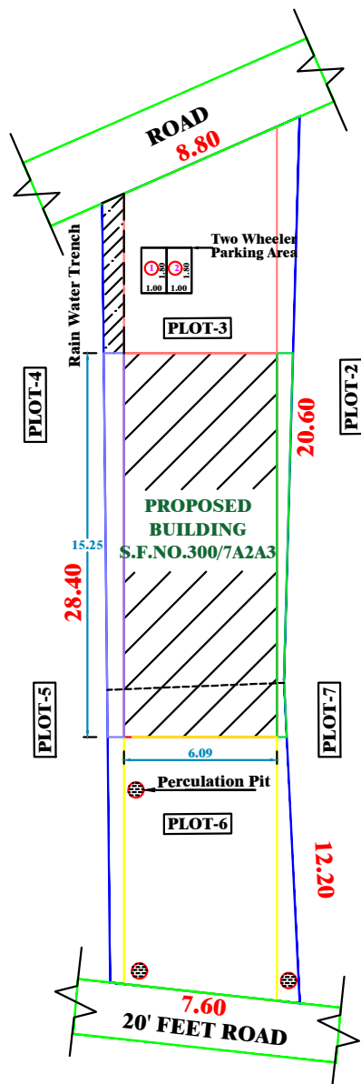
SITE PLAN - (SCALE 1:500)
