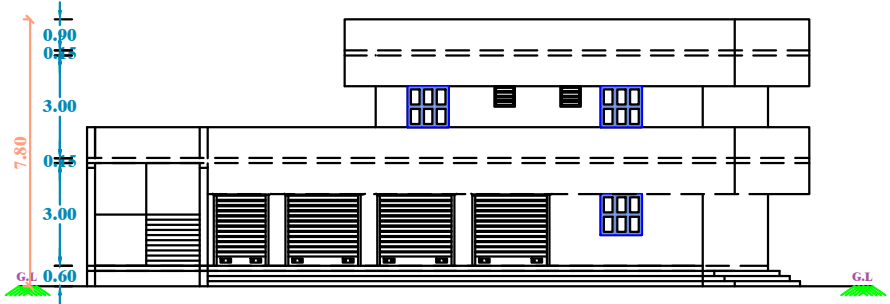
ELEVATION
