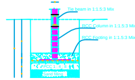
CROSS SECTION (P.V. P.C.)
