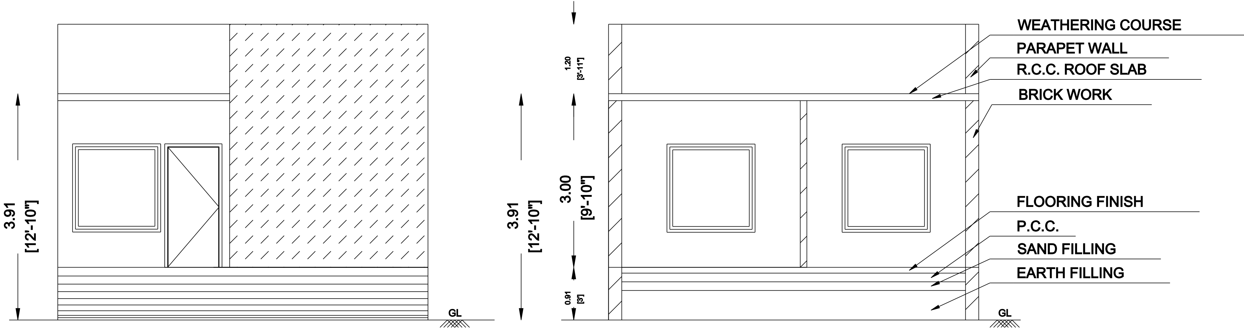
ELEVATION
