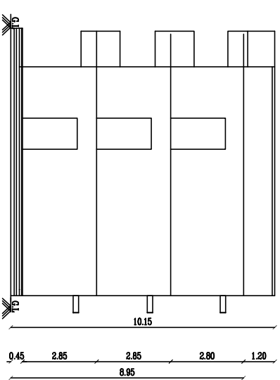
ELEVATION
