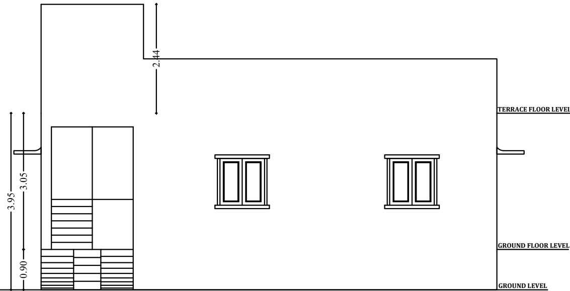
ELEVATION
