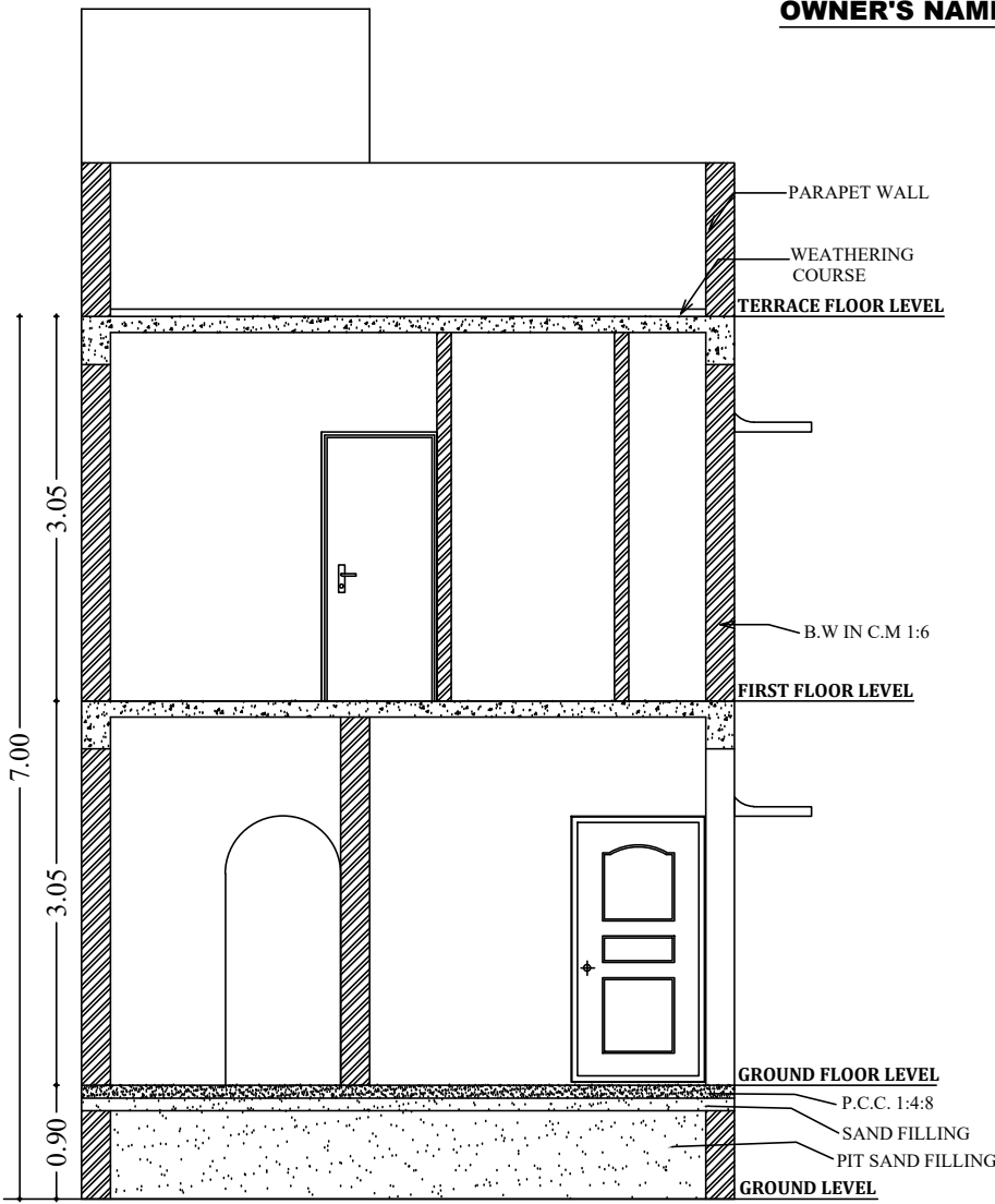
SECTION A-A'
