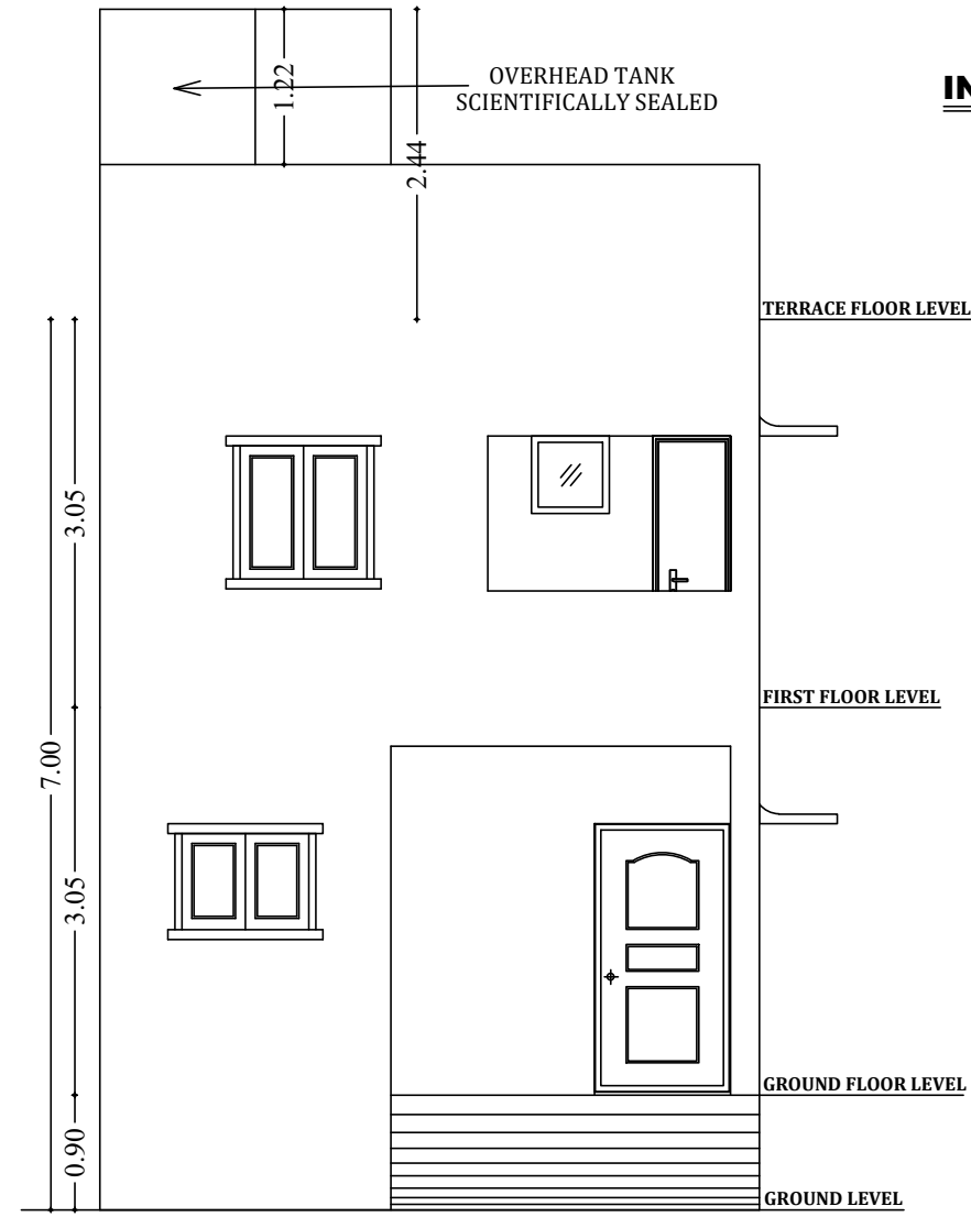
ELEVATION
