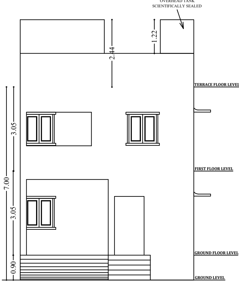
ELEVATION
