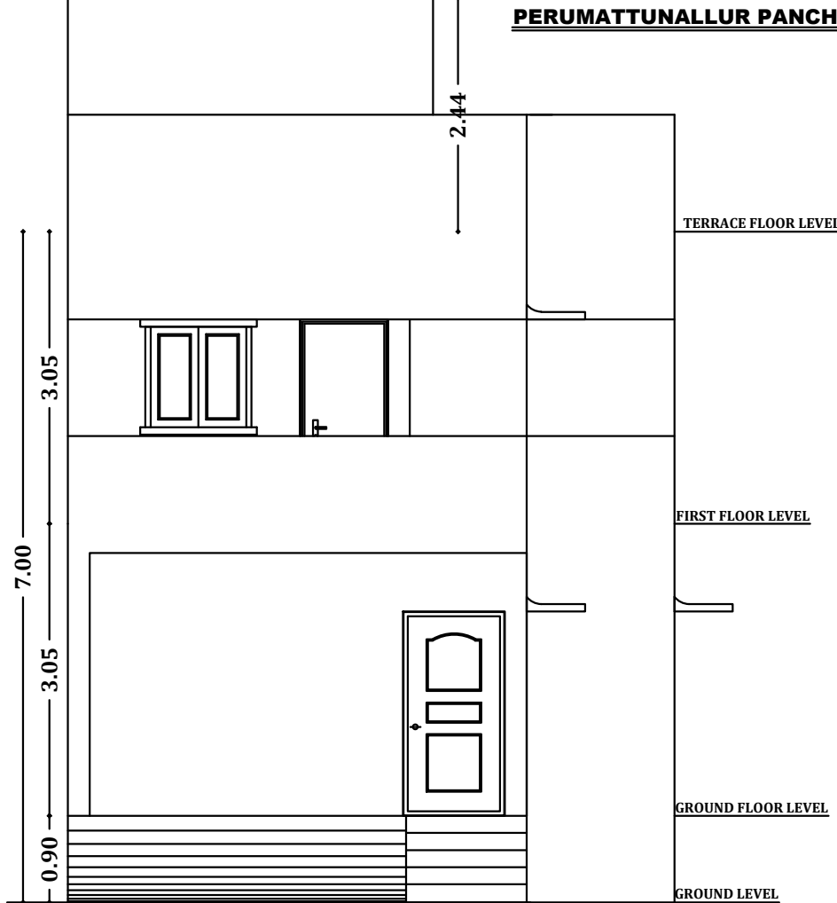
ELEVATION
