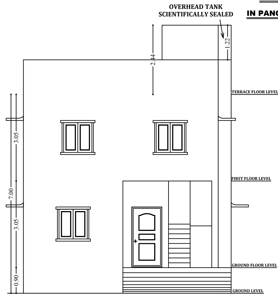
ELEVATION
