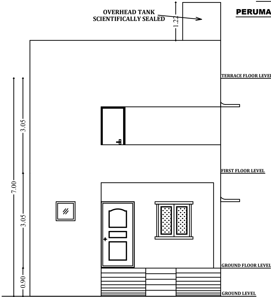
ELEVATION
