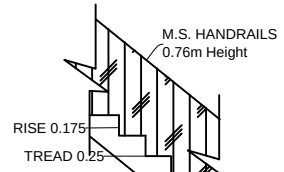
STAIRCASE DETAILS SCALE: 1:20
