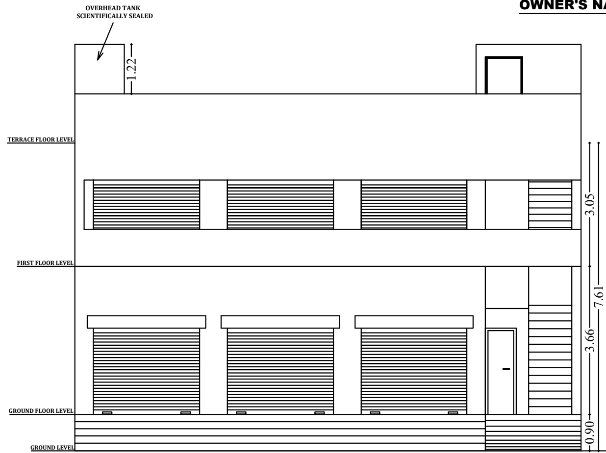
ELEVATION
