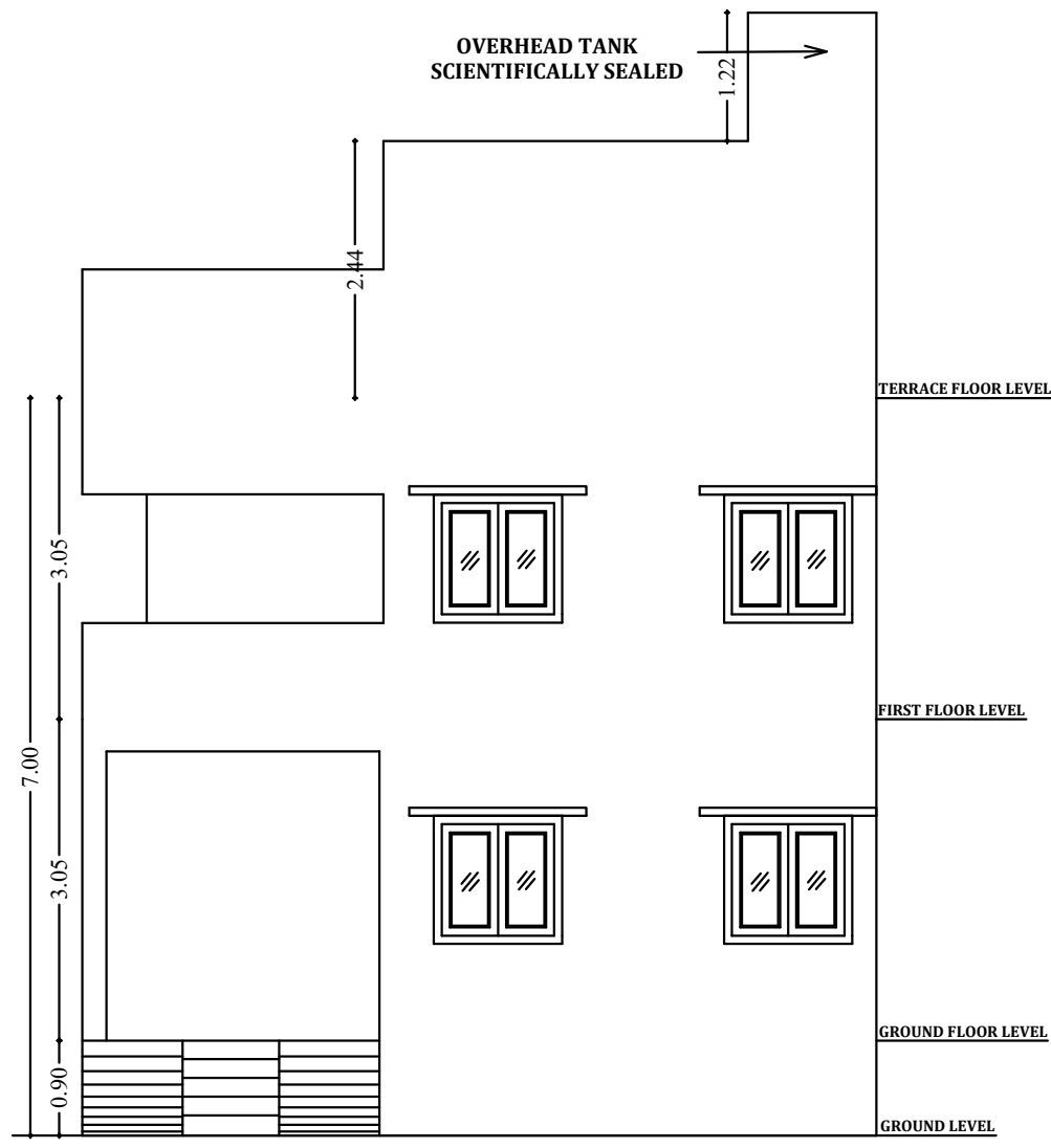
ELEVATION
