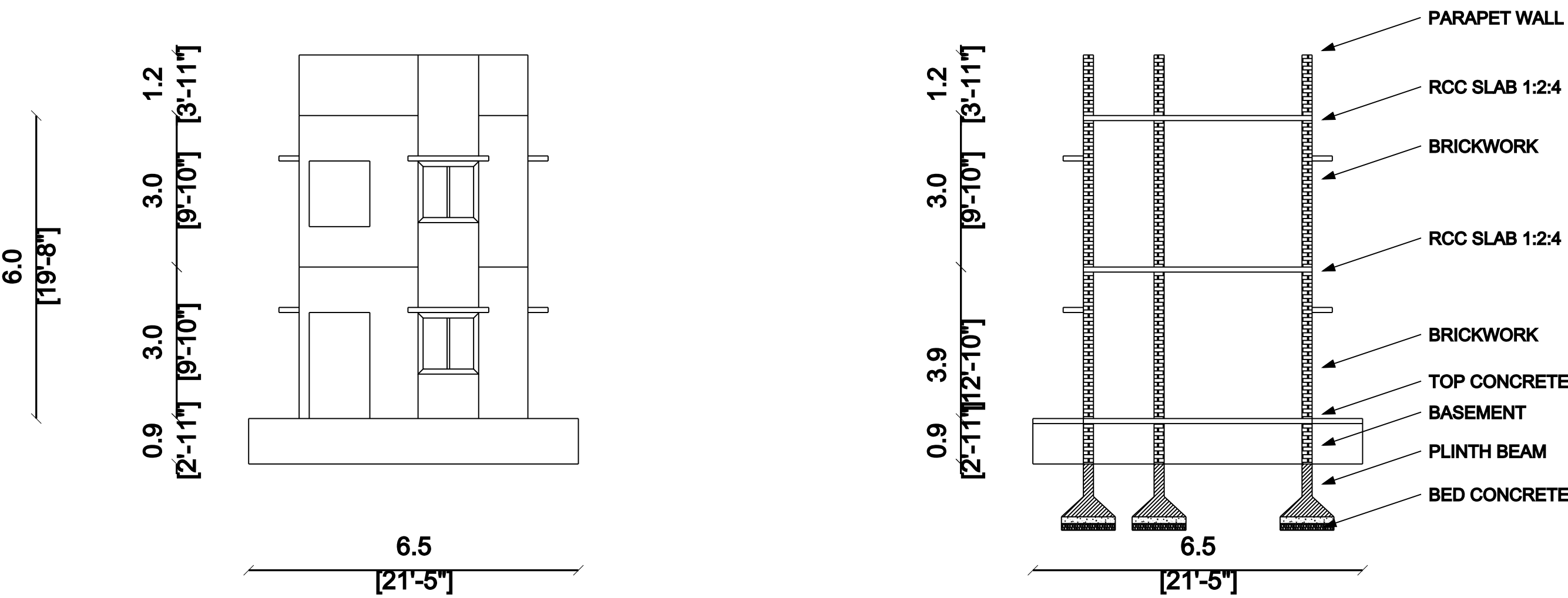
ELEVATION
