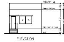
ELEVATION
