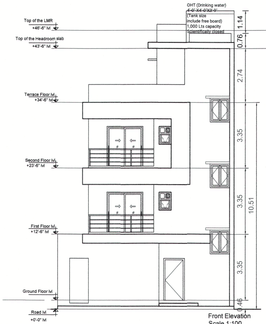
ELEVATION
