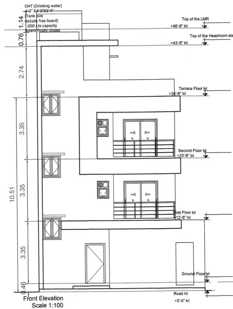
ELEVATION
