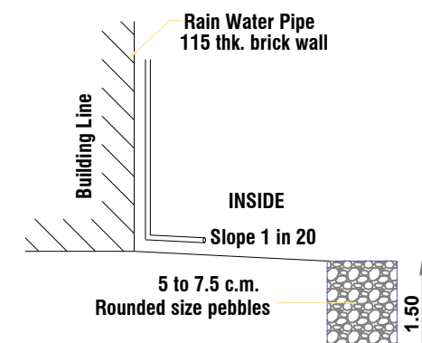
RWH -TRENCH
